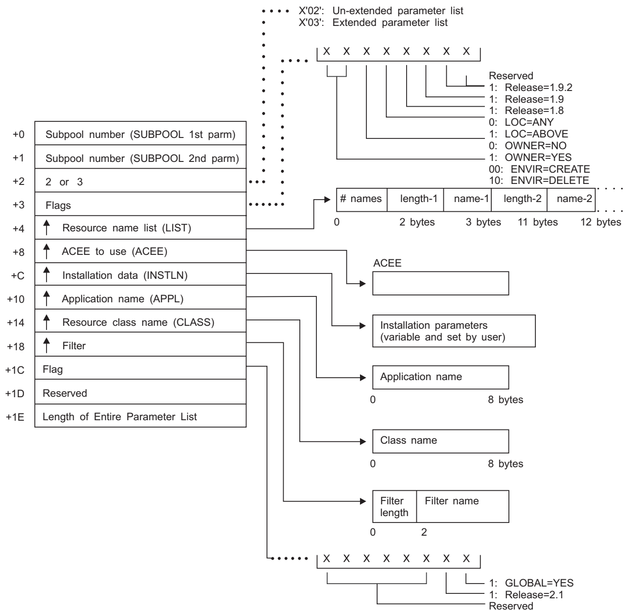
Figure 33. LIST Service Parameter List
