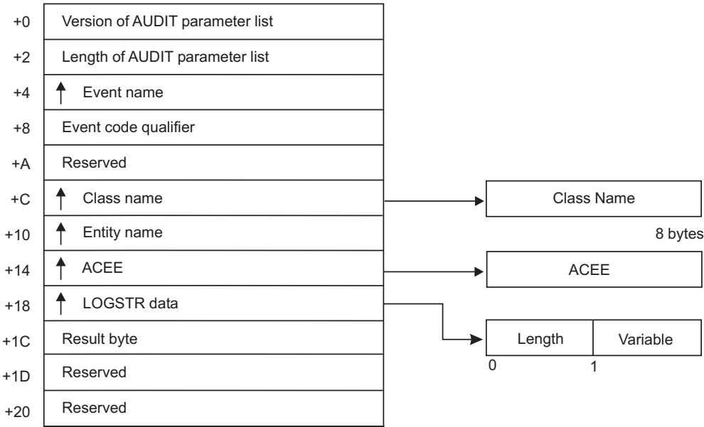
Figure 27. AUDIT Service Parameter List
